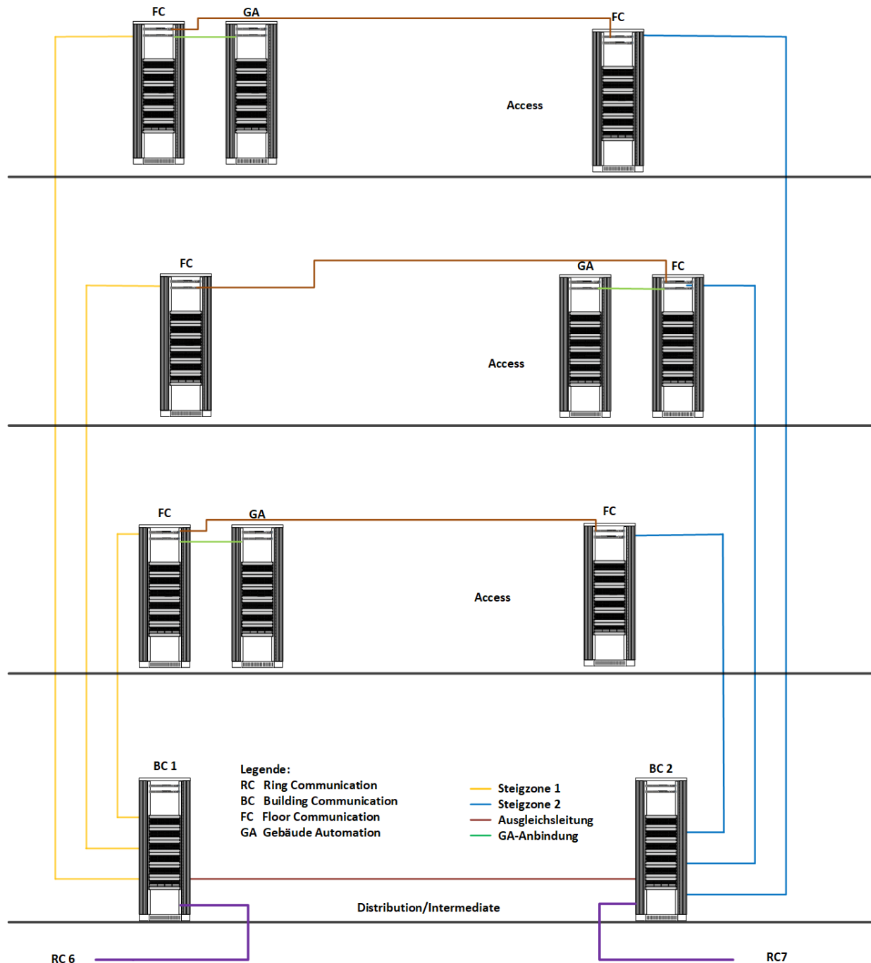
Abbildung 2 Steigzonenerschliessung
