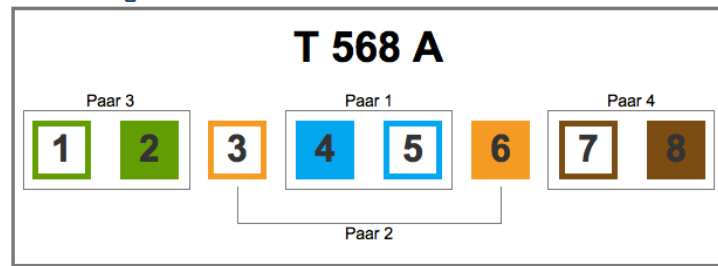
Abbildung 5 EIA/TIA-568
