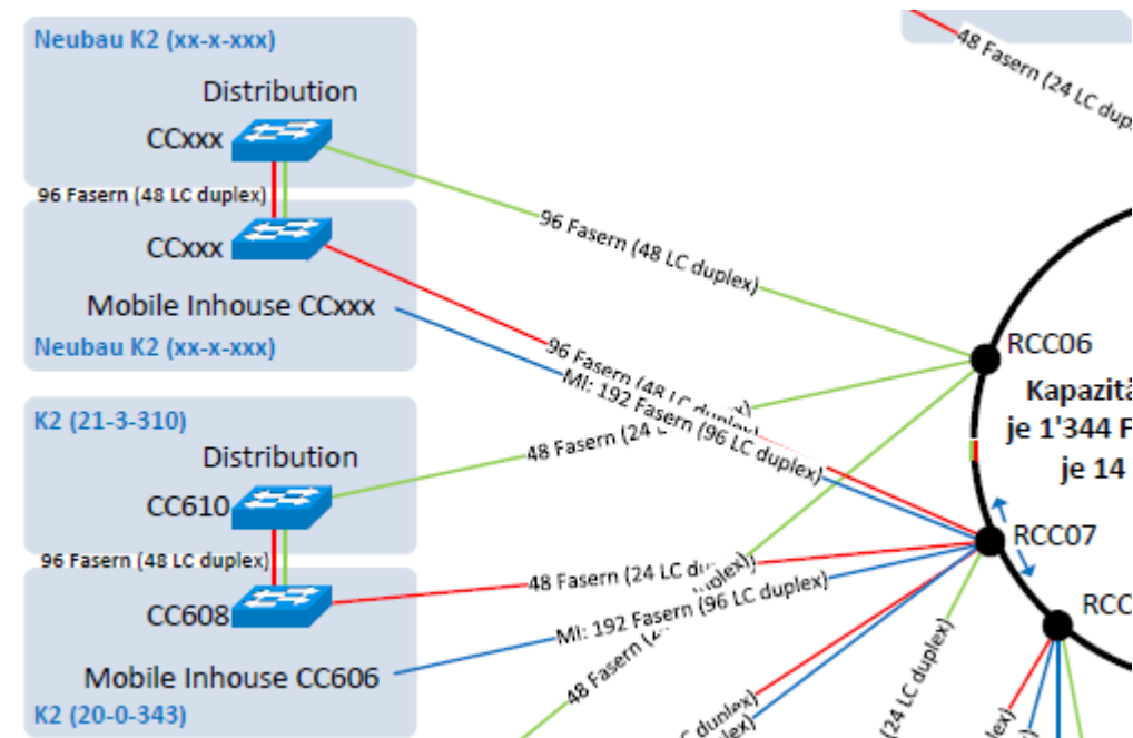
Abbildung 1 Gebäudeerschließung
